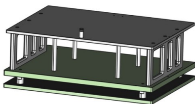
Andruckplatte (AP)
